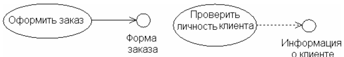
Рис. 23 Графическое изображение взаимосвязей интерфейсов с вариантами использования
