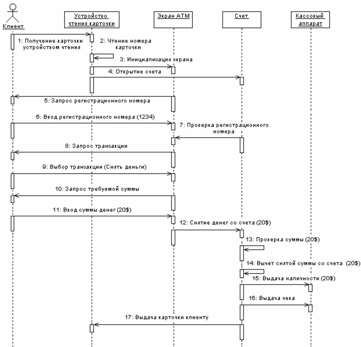
Рис. 34 Диаграмма последовательности для снятия клиентом 20$
