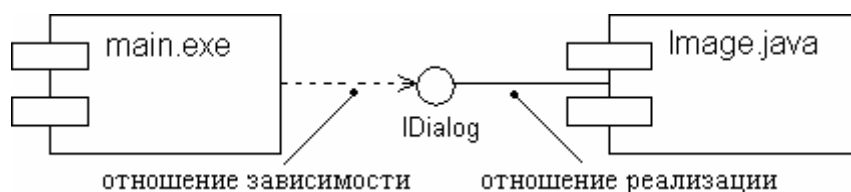
Рис. 65. Фрагмент диаграммы компонентов с отношением зависимости
