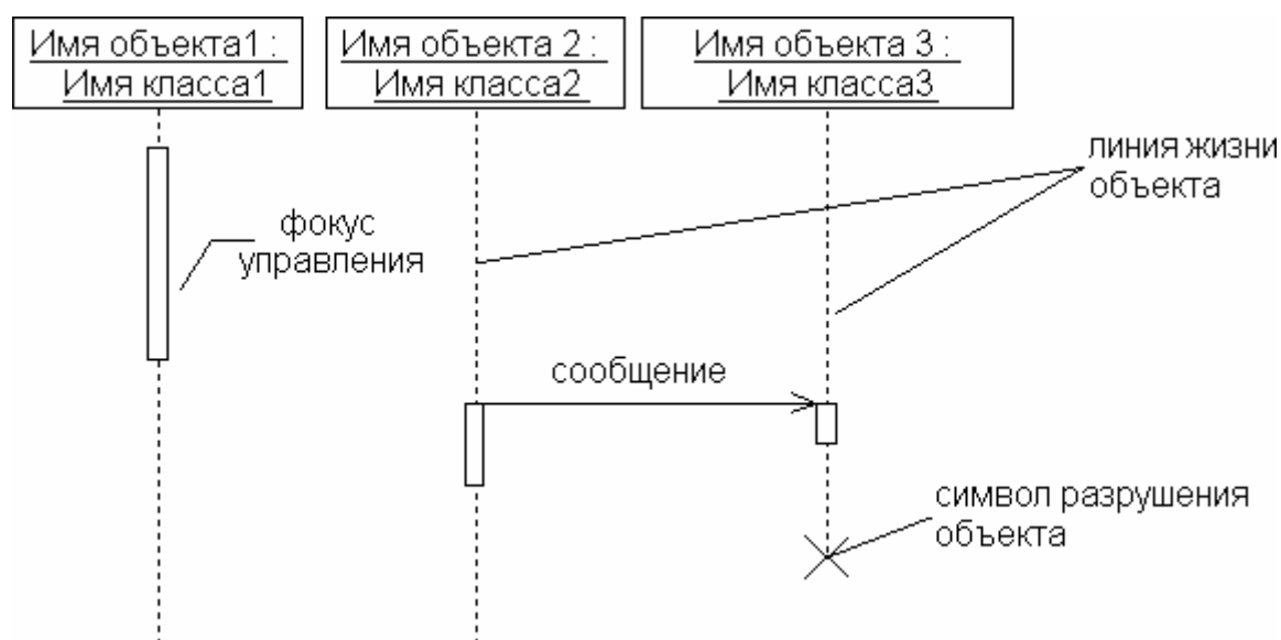
Рис. 31 Графические примитивы диаграммы последовательности
