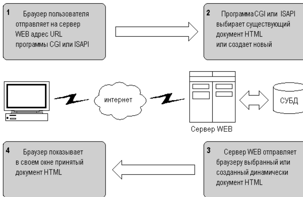
Рис. 1. Взаимодействие клиентского браузера и программного расширения
