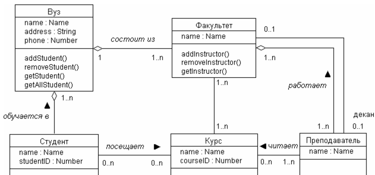
Рис. 51 Диаграмма классов для информационной системы ВУЗа
