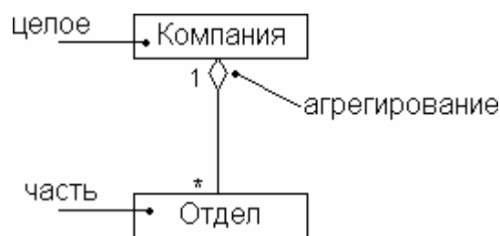
Рис. 15 Агрегирование
