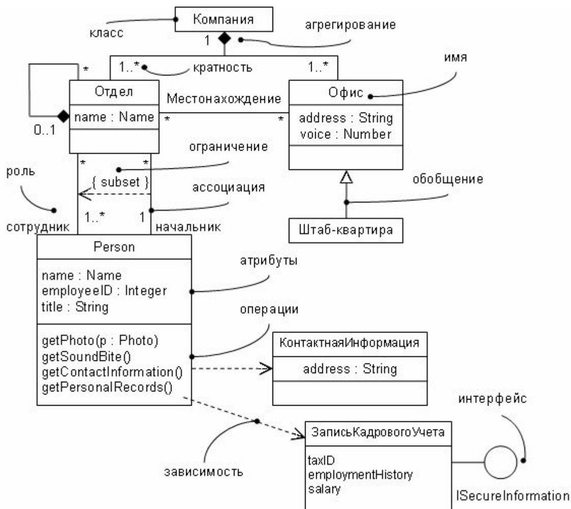
Рис. 52 Диаграмма классов
