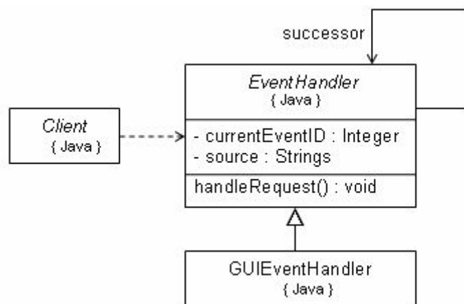
Рис. 50 Прямое проектирование
