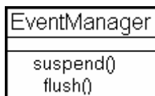
Рис. 7 Активный класс
