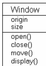
Рис. 3 Классы
