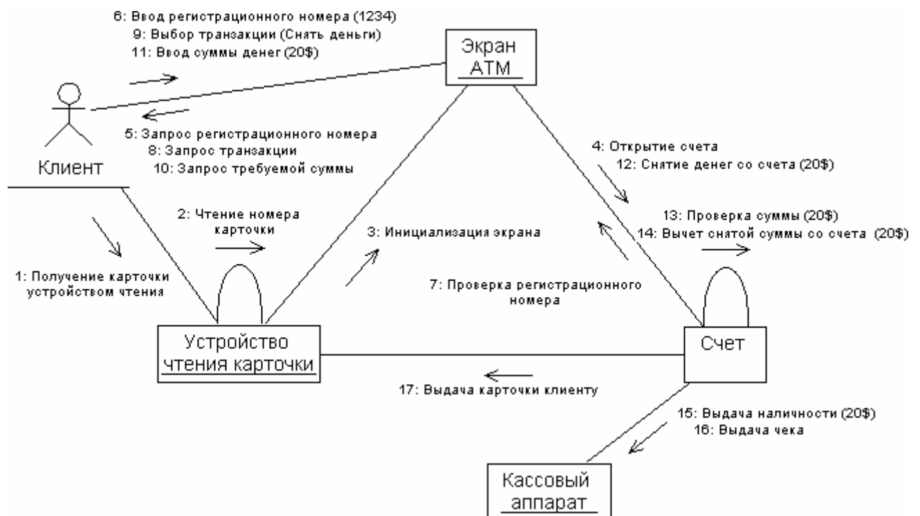
Рис. 39 Диаграмма кооперации для снятия клиентом 20$
