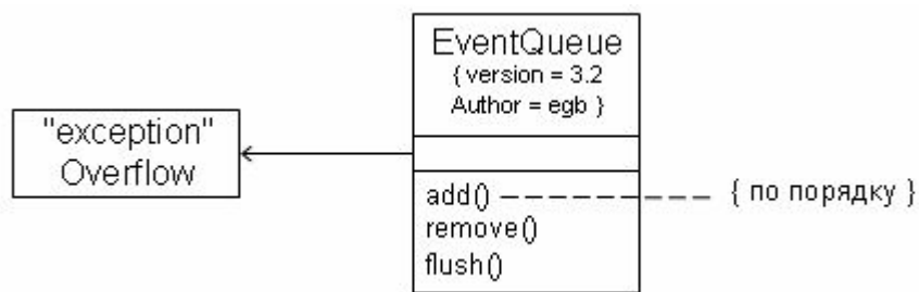
Рис. 48 Помеченное значение
