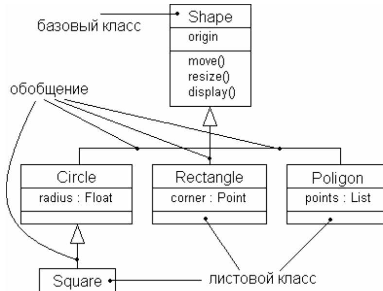
Рис. 17 Обобщение
