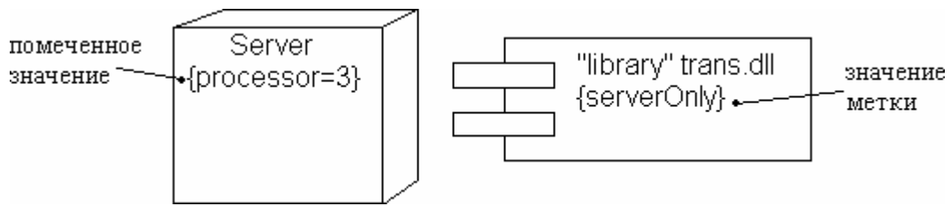
Рис. 68 Помеченные значения
