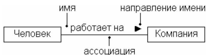
Рис. 16 Имена ассоциаций
