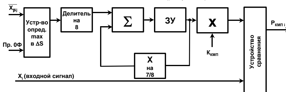
Рисунок 1 – Структурная схема устройства компенсации местных предметов
