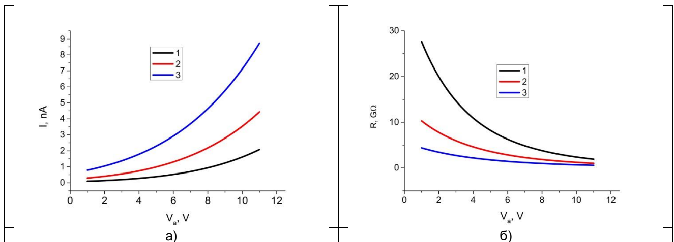
Рисунок 2 – Анодная характеристика (а) и внутренне сопротивление (б) нанотриода: 1 - V_g= 10,2 В, 2 - V_g= 11,0 В, 3 - V_g= 11,8 В
