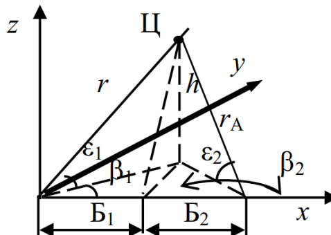
Рис. 1 – Угломерный метод определения местоположения объектов
