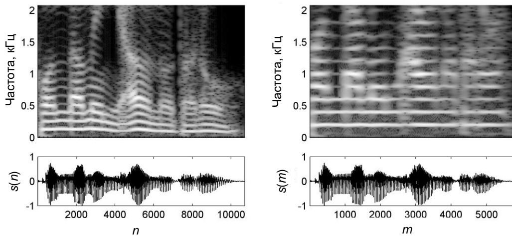
Рисунок 2 – Результат передискретизации согласованной с частотой основного тона
