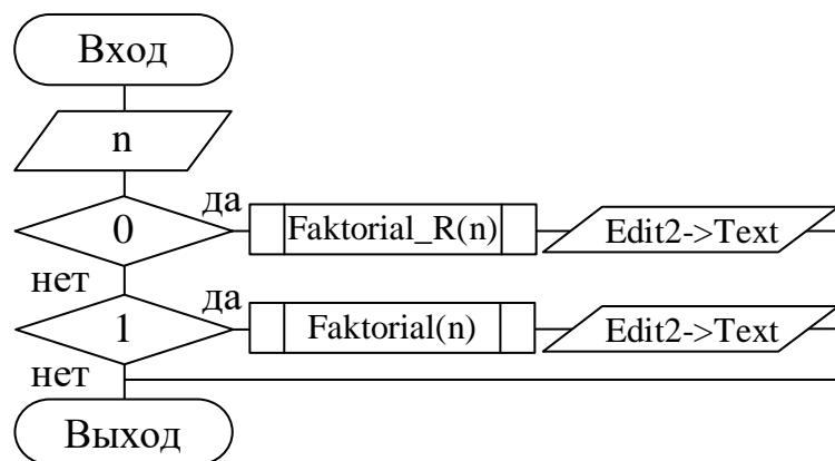
Рис. 1.1. Блок – схема вызова рекурсивной и нерекурсивной функции
