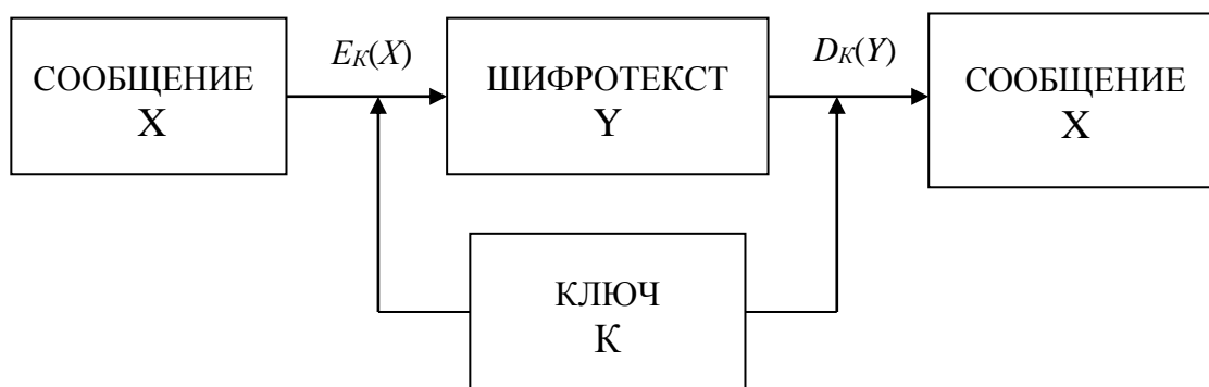
Рис. 3.1. Симметричное шифрование
